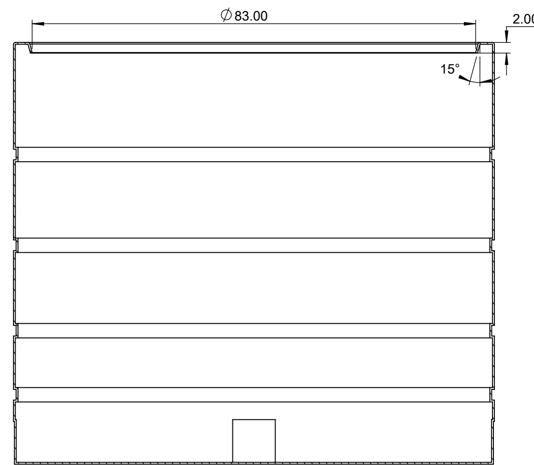
SECTION A-A
