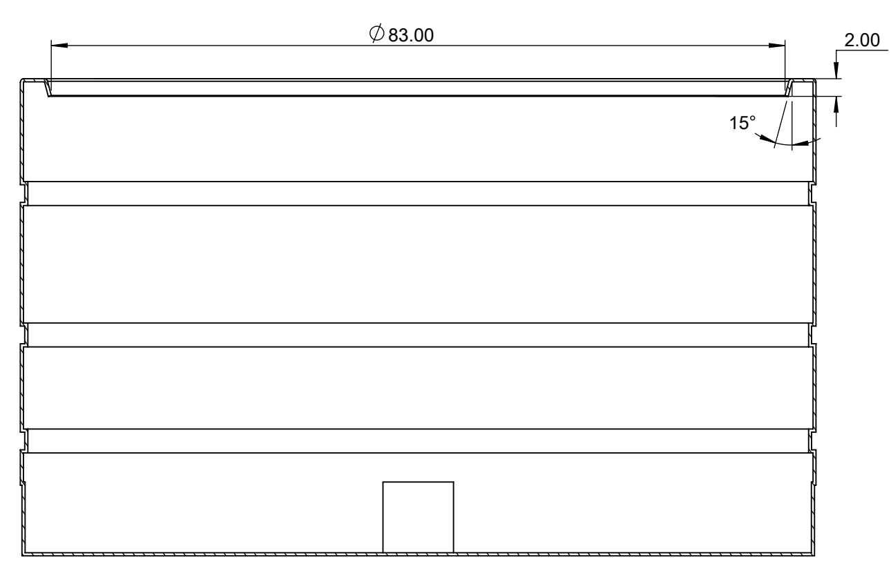
SECTION A-A
